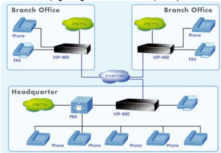
VIP-480 sử dụng trong mô hình kết nối điện thoại IP đa điểm
